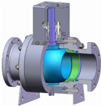
标准型 (NPS≥6)
