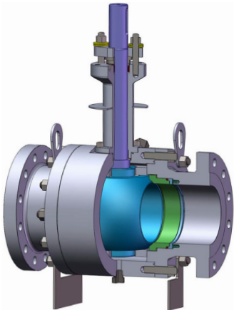
低温型
