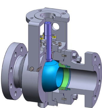
标准型 (NPS≤4)
